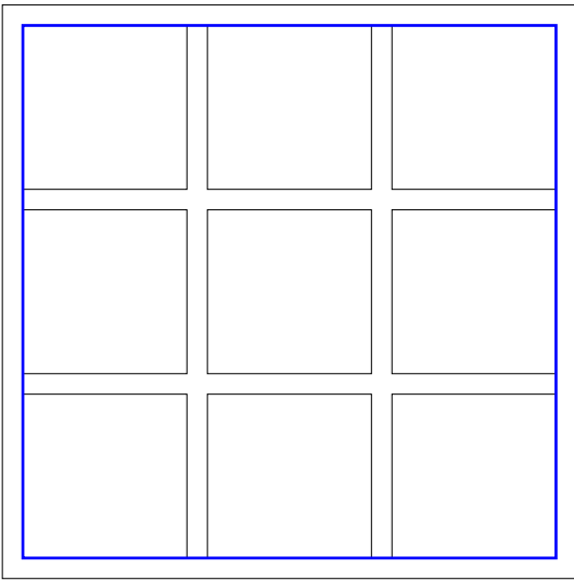
(default)
