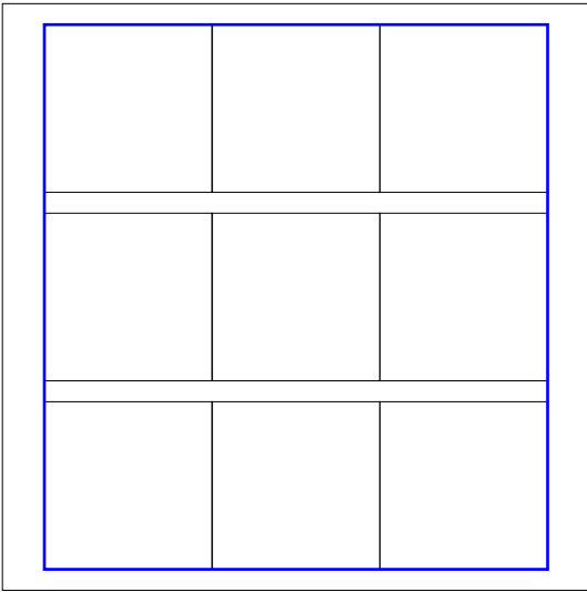
xpack => 'center'
